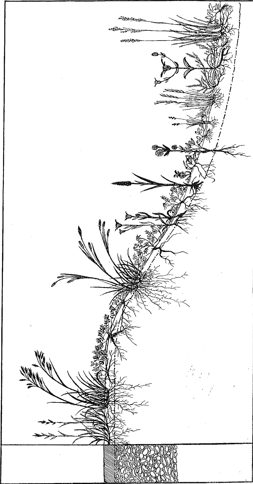
Abb. 5. Vegetationsprofil einer Bromus erectus - Carex sempervirens -reichen Grasflur im Kirchseegebiet. Brachypodium pinnatum , Bromus erectus , Polygala chamaebuxus , Teucrium montanum , Globularia cordifolia , Carex sempervirens , Hippocrepis comosa , Buphthalmum salicifolium , Gymnadenia conopsea , Brunella grandiflora , Trifolium montanum , Potentilla Tormentilla , Siegingia decumbens , Nardus stricta , Calluna vulgaris , Arnica montana und Molinia caerulea .
