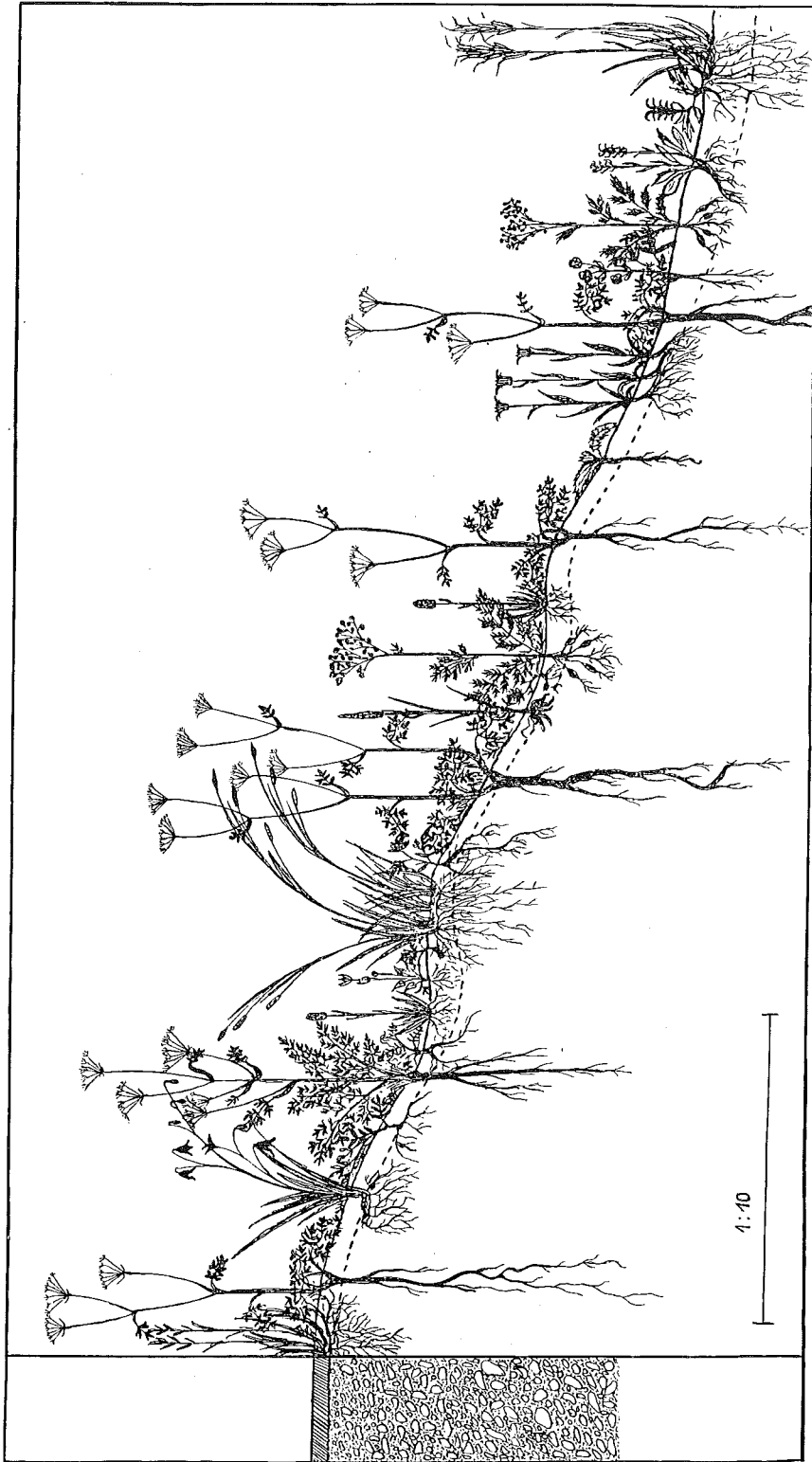
Abb. 4. Vegetationsprofil. Peucedanum Oreoselinum - Anthericum ramosum -reiche Feldschicht des Steppenheide-Eichenwaldes auf der Oberwarngauer Endmoräne (Osterwarngau). Brachypodium pinnatum , Peucedanum Oreoselinum , Anthericum ramosum , Polygala Chamaebuxus , Seseli Libanotis , Hippocrepis comosa , Tofieldia calyculata , Parnassia palustris , Carex sempervirens , Antyllus Vulneraria , Gymnadenia conopsea , Filipendula hexapetala , Carlina acutis , Buphthalmum salicifolium , Trifolium montanum , Stachys officinalis , Prunella grandiflora , Avena pratensis .
